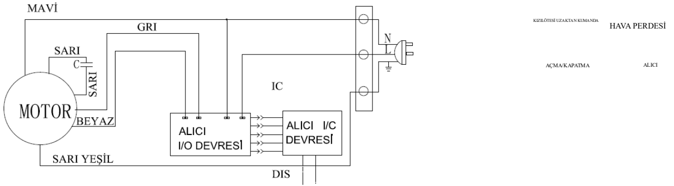
ÇİFT HIZ INFRARED UZAKTAN KUMANDA TEL BAĞLANTI ŞEMASI
